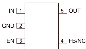
SOT23-5
