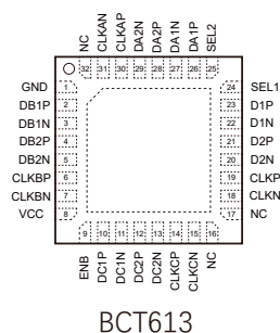
QFN4x4-32L
