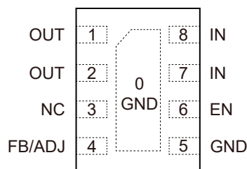
DFN1.6x1.2-8L
