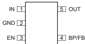
SOT23-5 SC70-5
