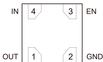
DFNFC1x1-4L
