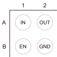
WLCSP-4L
