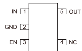
SOT23-5
