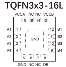
BCT0104
