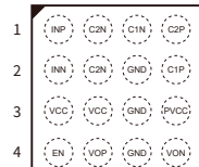
BCT8937A/BCT89317A BCT89318A
