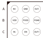
BCT8013
