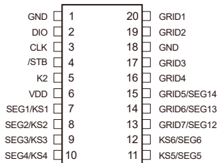
BCT3620B
