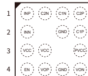
BCT8327
