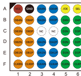
FO-36L
