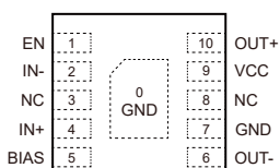
BCT8996
