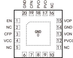
BCT8933B
