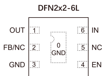
BCT2057/BCT2186L
