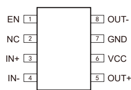
BCT8005
