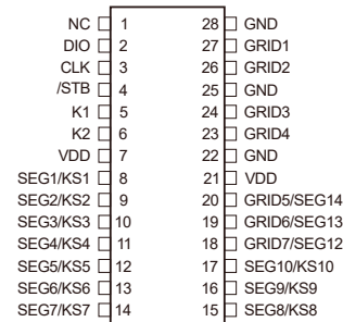
BCT3628X/BCT1628X BCT3628A
