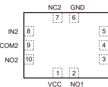
BCT4223
