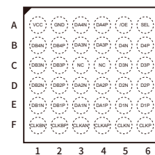
FO-36L
