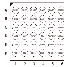
FO-36L
