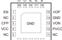
BCT8933B
