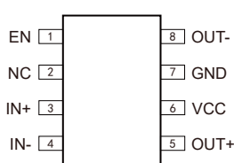
BCT8005
